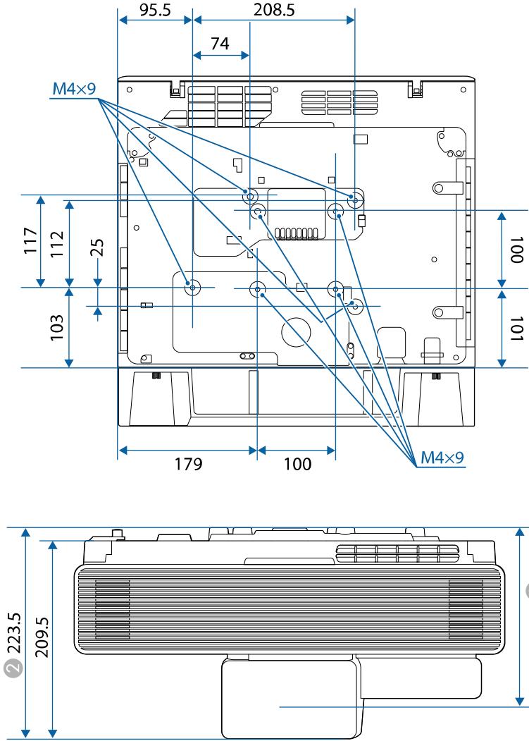
EB-1485Fi/EB-1480Fi:
