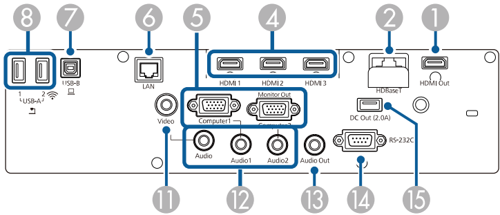
EB-805F/EB-800F
