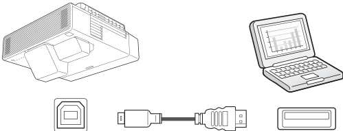
USB-B
